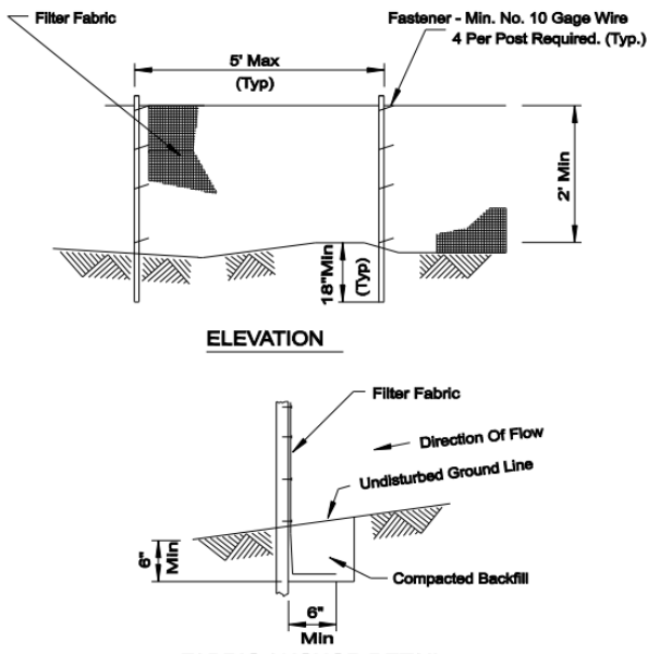
Standard IL Drawing:
